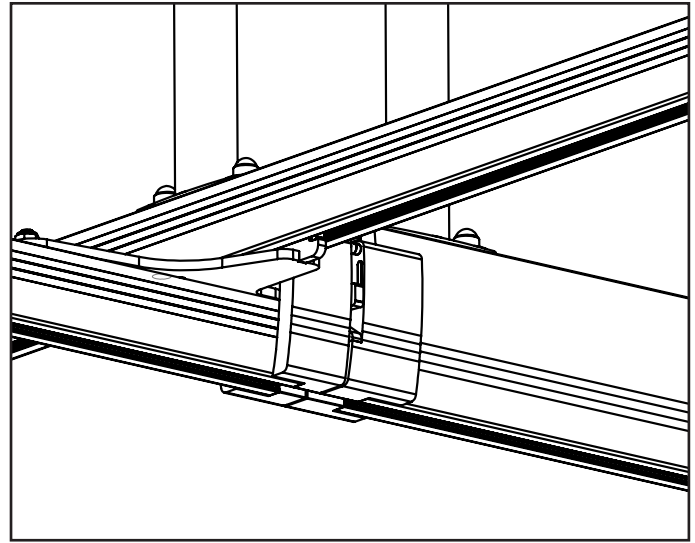
Přesun – připojená příčná spojka
