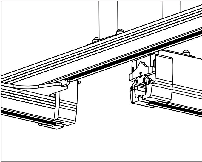
Přesun – odpojená příčná spojka
