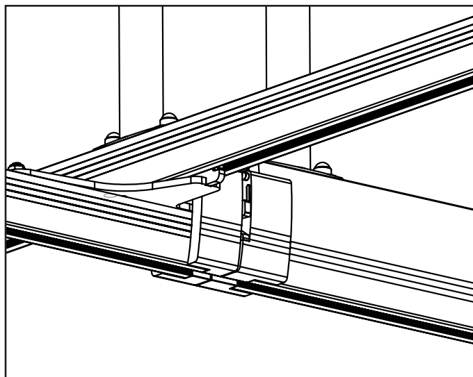
Prenos – priključena prenosna spojka
