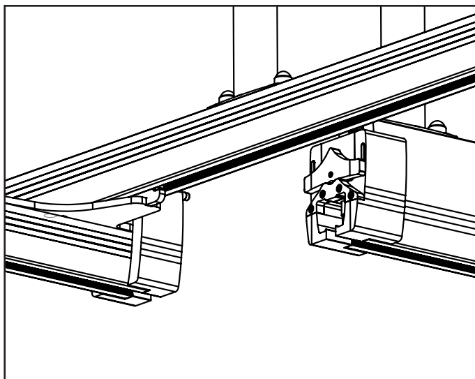
Prenos – odklopljena prenosna spojka
