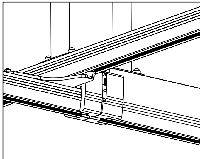
Trasferimento: raccordo di traversale collegato
