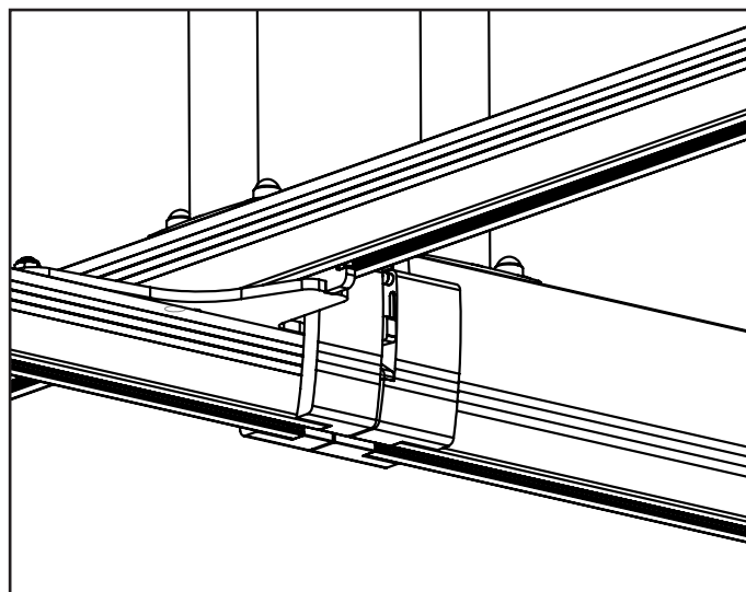
Forflytning – tilkoblet traverskobling
